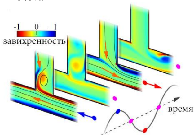
Рис. 2. Моделирование потоков воздуха при пульсации в Т-образном соединении
