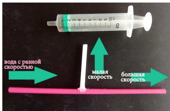
Рис. 3. Приборы и схема простого эксперимента: шприц с поршнем, склеенная трубочка.
