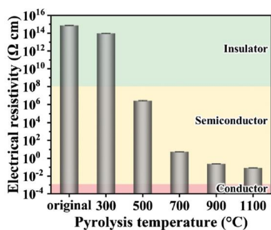
Рис. 5. Электрическое сопротивление исходной хитиновой бумаги и углеродных наноматериалов, полученных в результате пиролиза.
